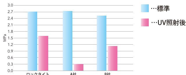
皮膜物性試験:引張速度100mm/minで、最大強度を測定。(23℃50%rhにて、7日間養生。55℃50%rhにて、メタルハライドランプ出力70mW・cm 2 で120時間照射) ※自社試験によるデータ 記載のデータは代表値です。性能を保証するものではありません。
