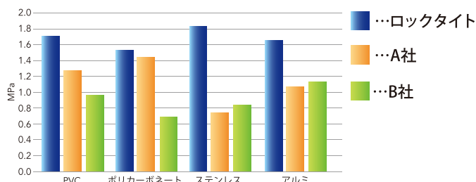
浸漬試験:引っぱりせん断強度を測定(23℃ 7日間養生+水3日間浸漬)
